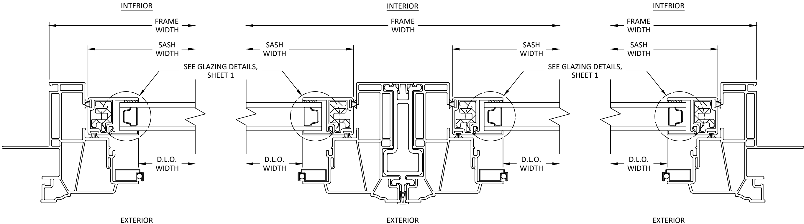
G 4 HORIZONTAL SECTION SASH JAMB
